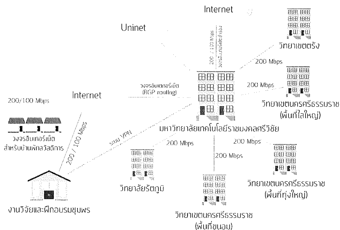
รูปแสดงวงจรเชื่อมต่อเครือข่ายของมหาวิทยาลัยเทคโนโลยีราชมงคลศรีวิชัย
