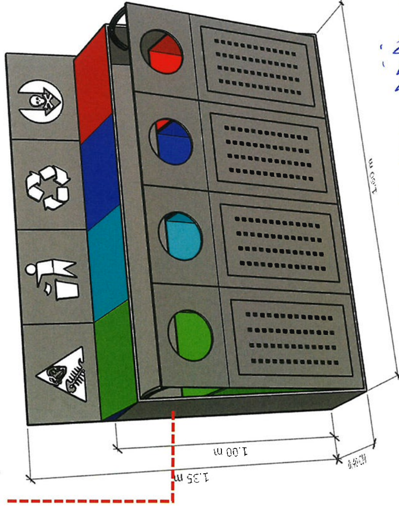
ภายนอกตู้ด้วยแผ่นคอมโพสิต ขนาดความหนา ๓-๔ มม. พร้อมทาสี
